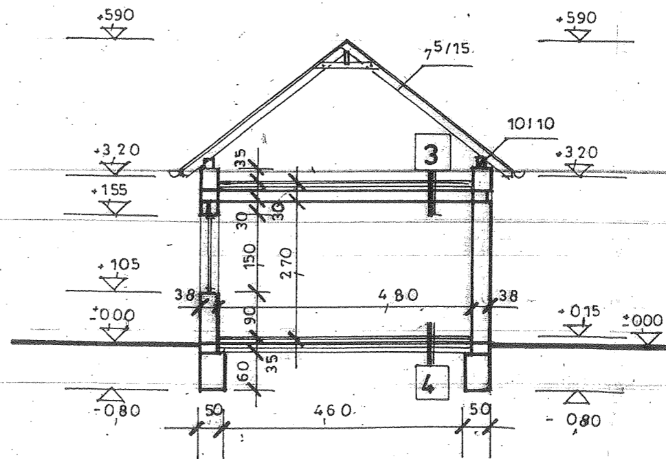
B - B METSZET
